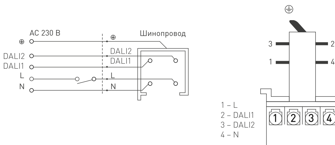
Рис. 2. Схема подключения
