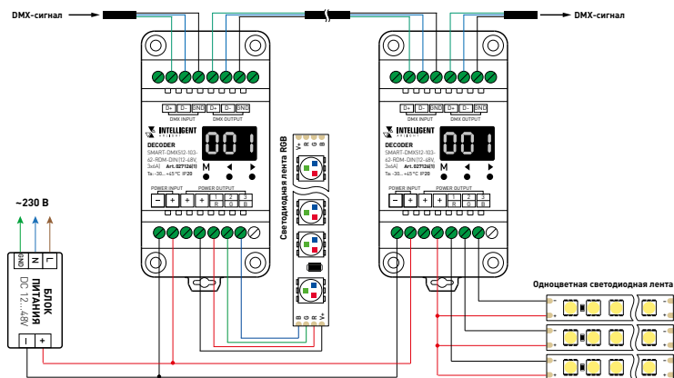
Рис. 1. Схема подключения декодера
