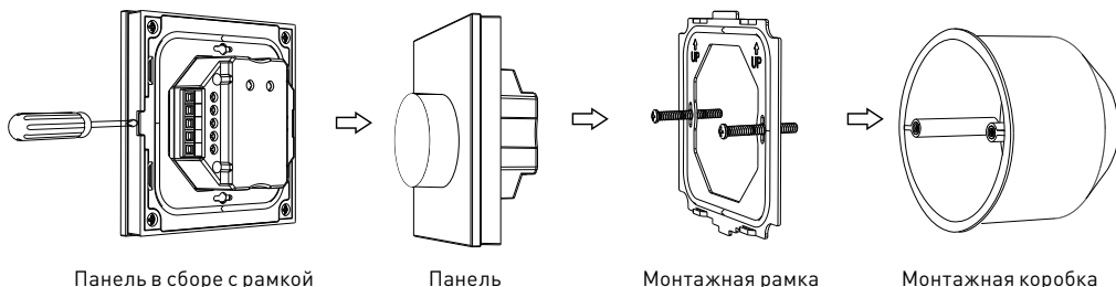
Рис. 4. Монтаж панели
