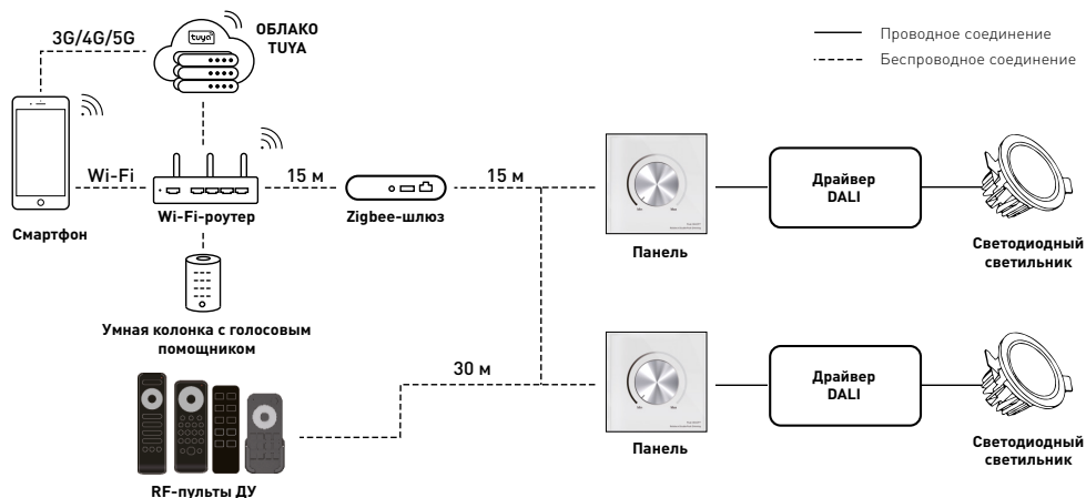
Рис. 3. Структурная схема построения системы
