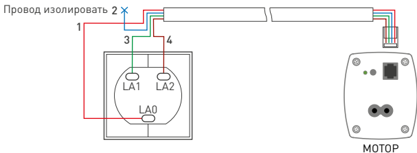
Рис. 1. Схема подключения
