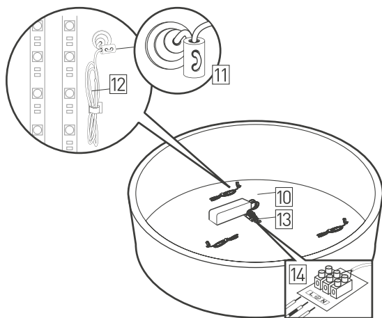
Рис. 2. Укладка кабеля
