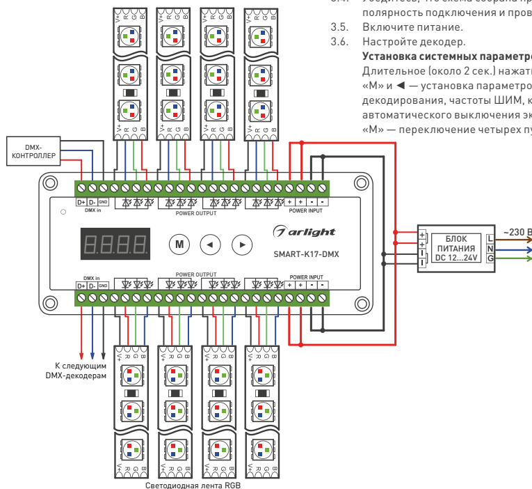
Рис. 1. Общая схема подключения декодера.
